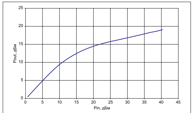
Рис. 12. Типовая зависимость выходной мощности от входной для ограничителя
